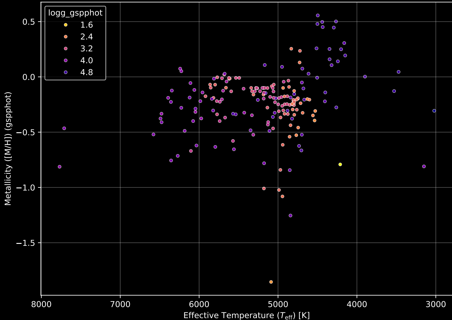
APOGEE DR17 Field: [010+60] Stellar Population Parameters (n= 190)
